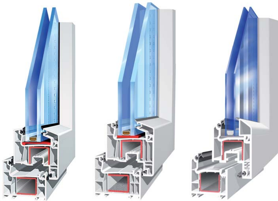
Профильная система Thermotech 752
