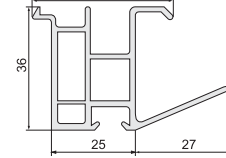
Арт. B77 (арт. VEKA -110.077)
