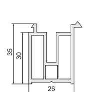
Арт. B26 (арт. VEKA -110.026)
