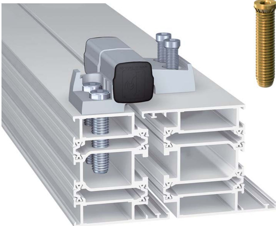
Новая петля Serie 60 AT (трехсекционное исполнение)
