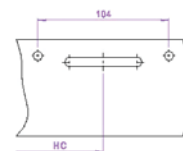
Пробивка паза
